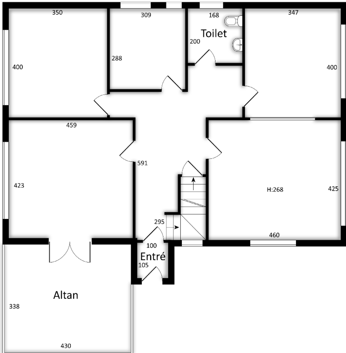
Stueplan
